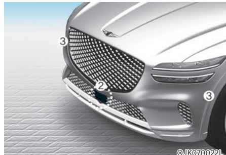
[1]: Frontkamera, [2]: Frontradar, [3]: Eckradar vorn (ausstattungsabhängig),
