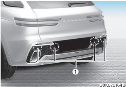
[1]: Ultraschallsensoren hinten
