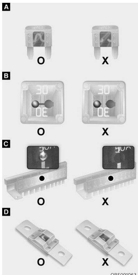
[A] : Type de lame, [B] : Type de cartouche, [C] : Type Multi, [D] : Type Midi O : Normal, X : Soufflé
