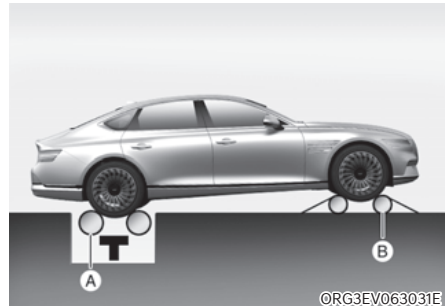
[A] : Rouleaux (compteur de vitesse), [B] : Rouleaux en roue libre temporaire
